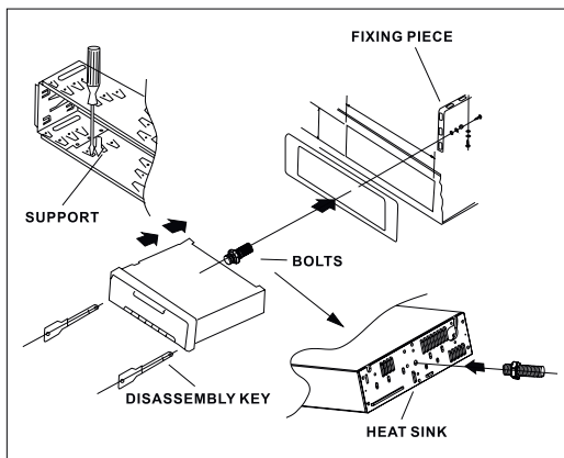
Installationsschema
