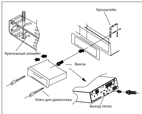
Схема инструкции
